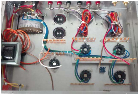
<電源一次、ヒーター、出力トランス2次側>
